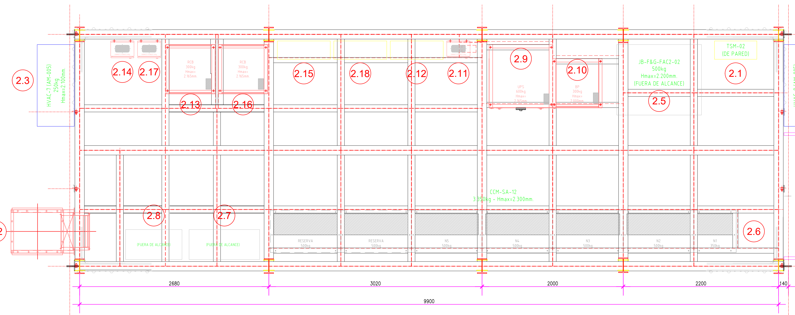
PLANTA PLATAFORMA PLT SEM-02 ESCALA 1:25
