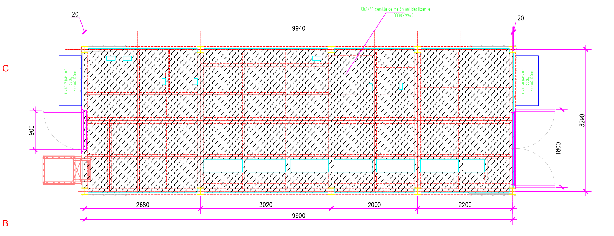
PLANTA CHAPA DE PISO PLATAFORMA PLT SEM-02 ESCALA 1:50
