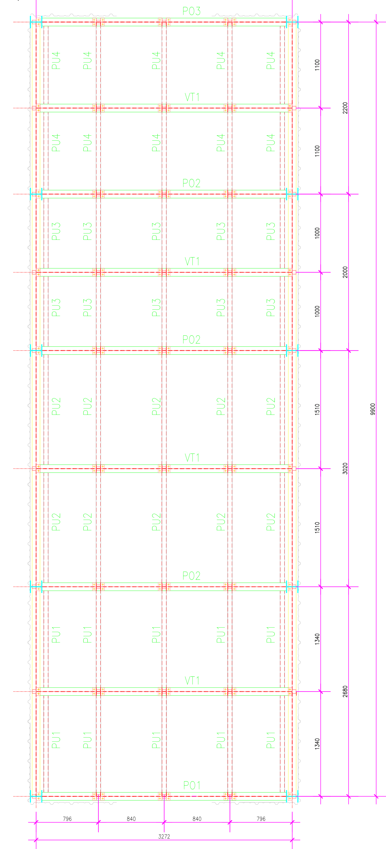
PLANTA PUNTALES ESCALA 1:25
