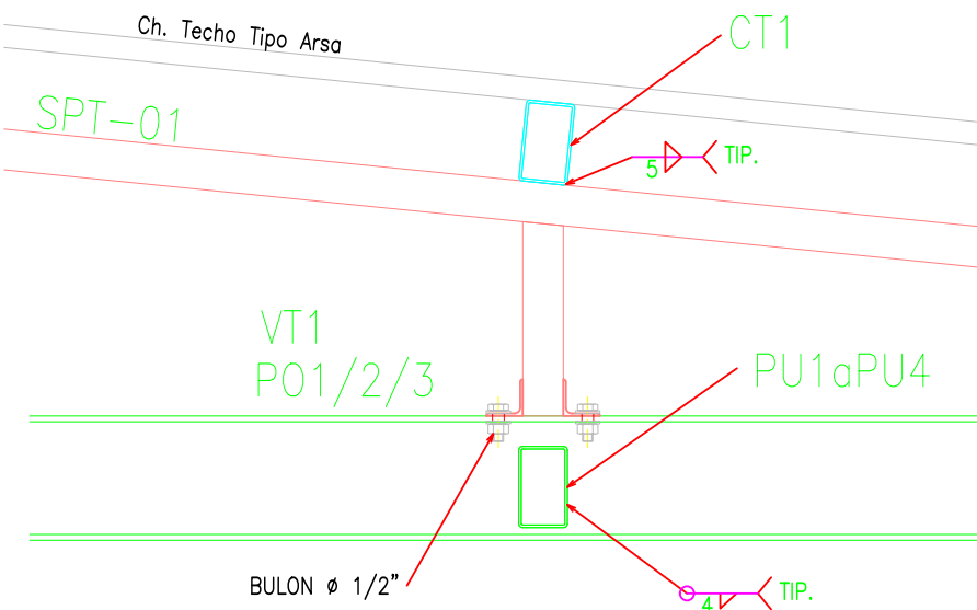
DET. 6 ESCALA 1:10
