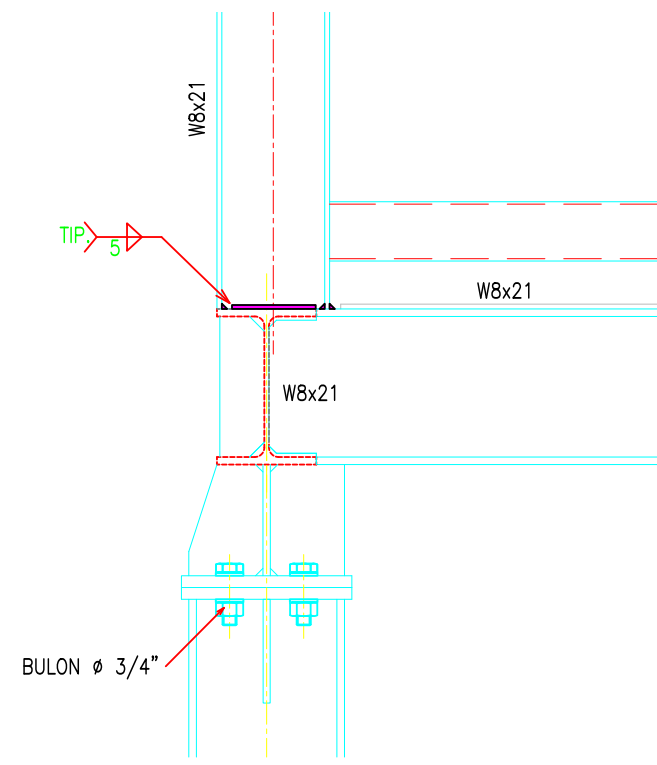
DET. 5 SOLD. NUDO INFERIOR ESCALA 1:10
