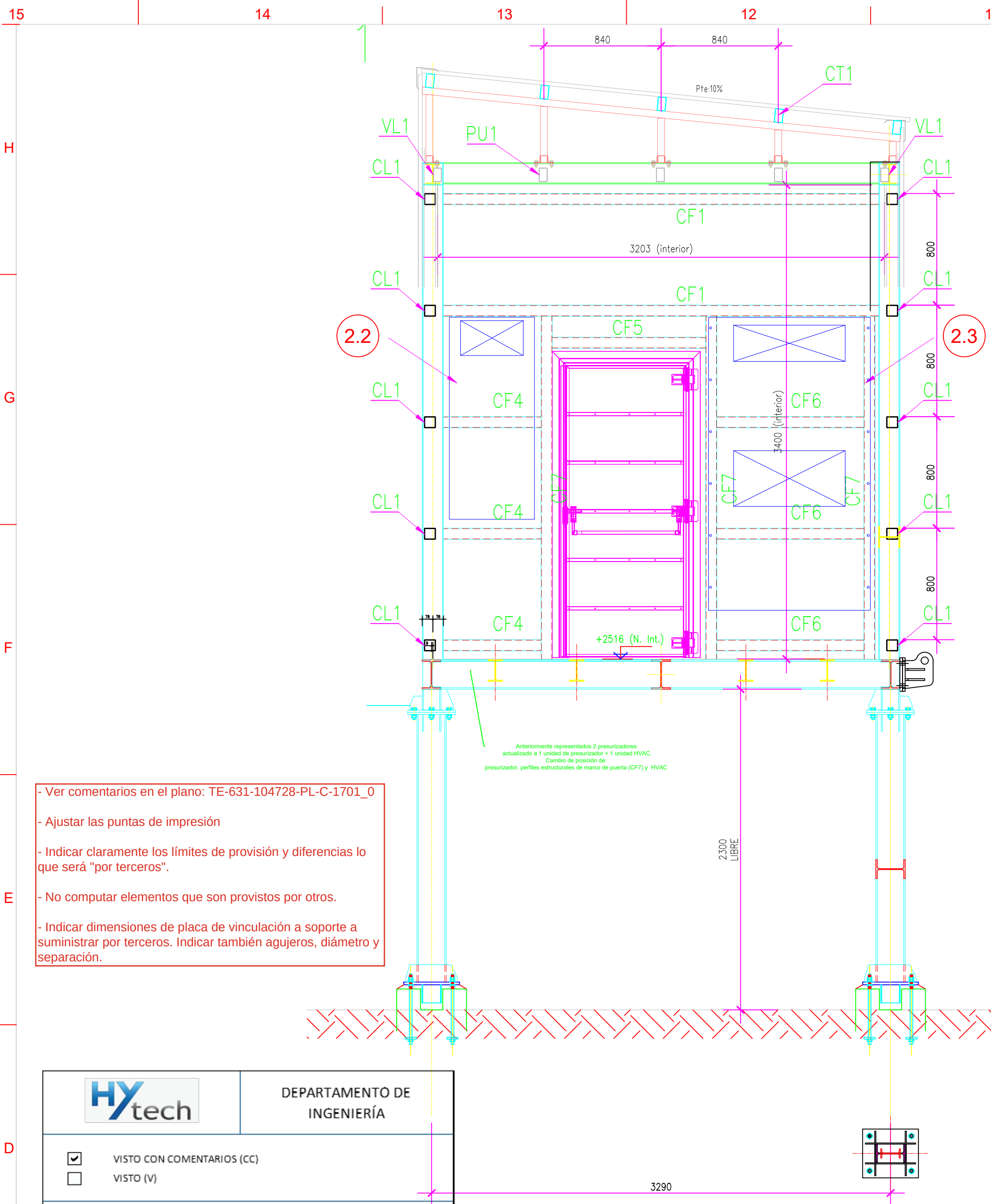
CORTE A-A SEM-02 ESCALA 1:25
