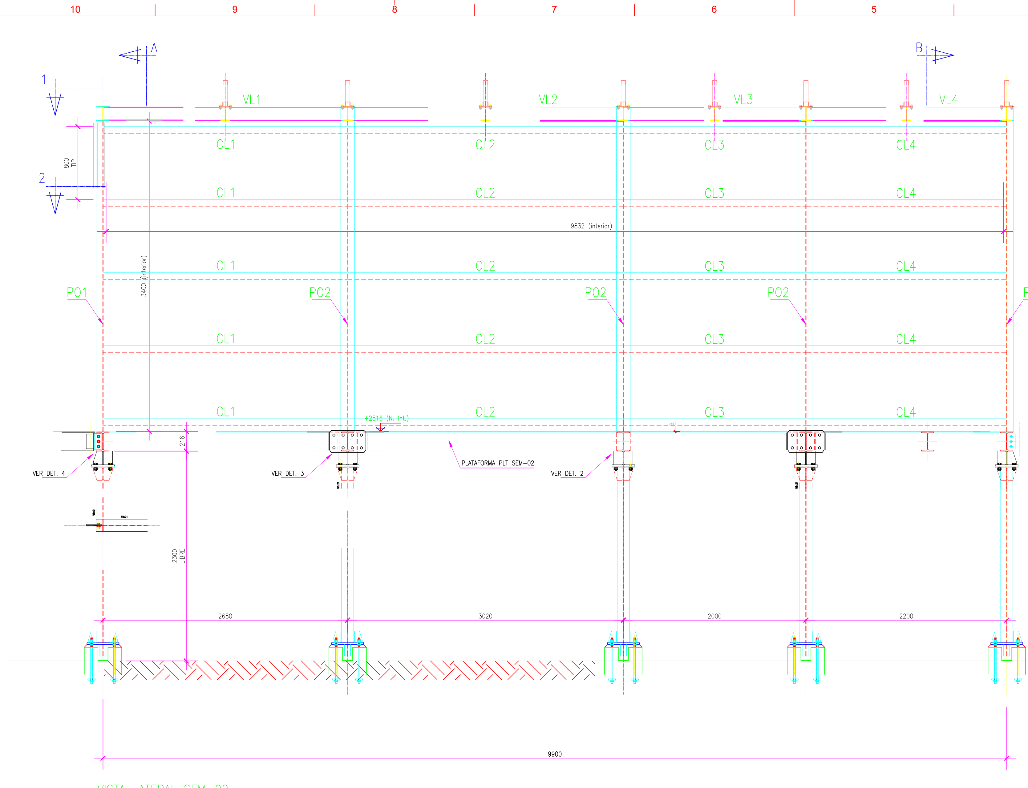
VISTA LATERAL SEM-02 ESCALA 1:25
